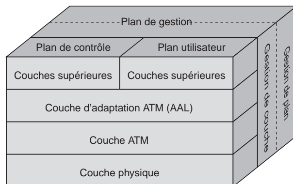
Figure 4.25 Couches de l'architecture UIT-T
