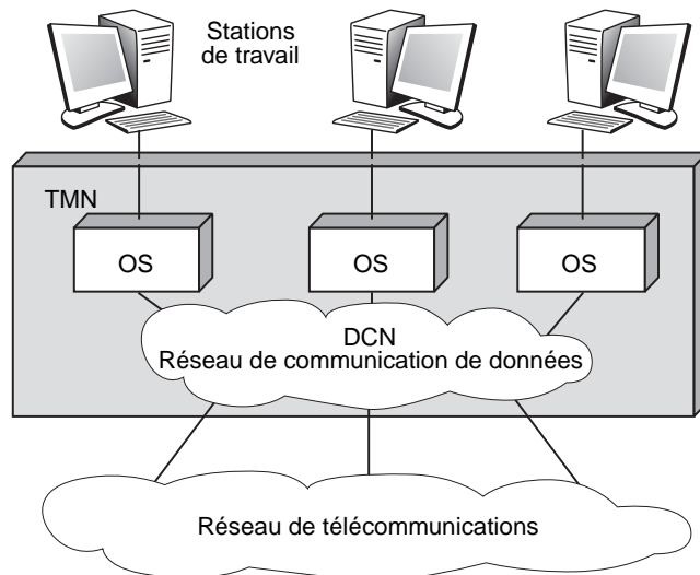
Figure 34.7 Architecture physique du TMN
