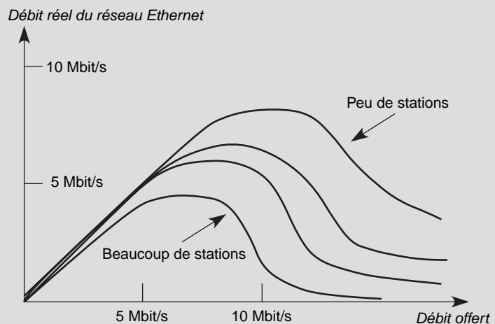
Figure 16.6 Performance du réseau Ethernet
