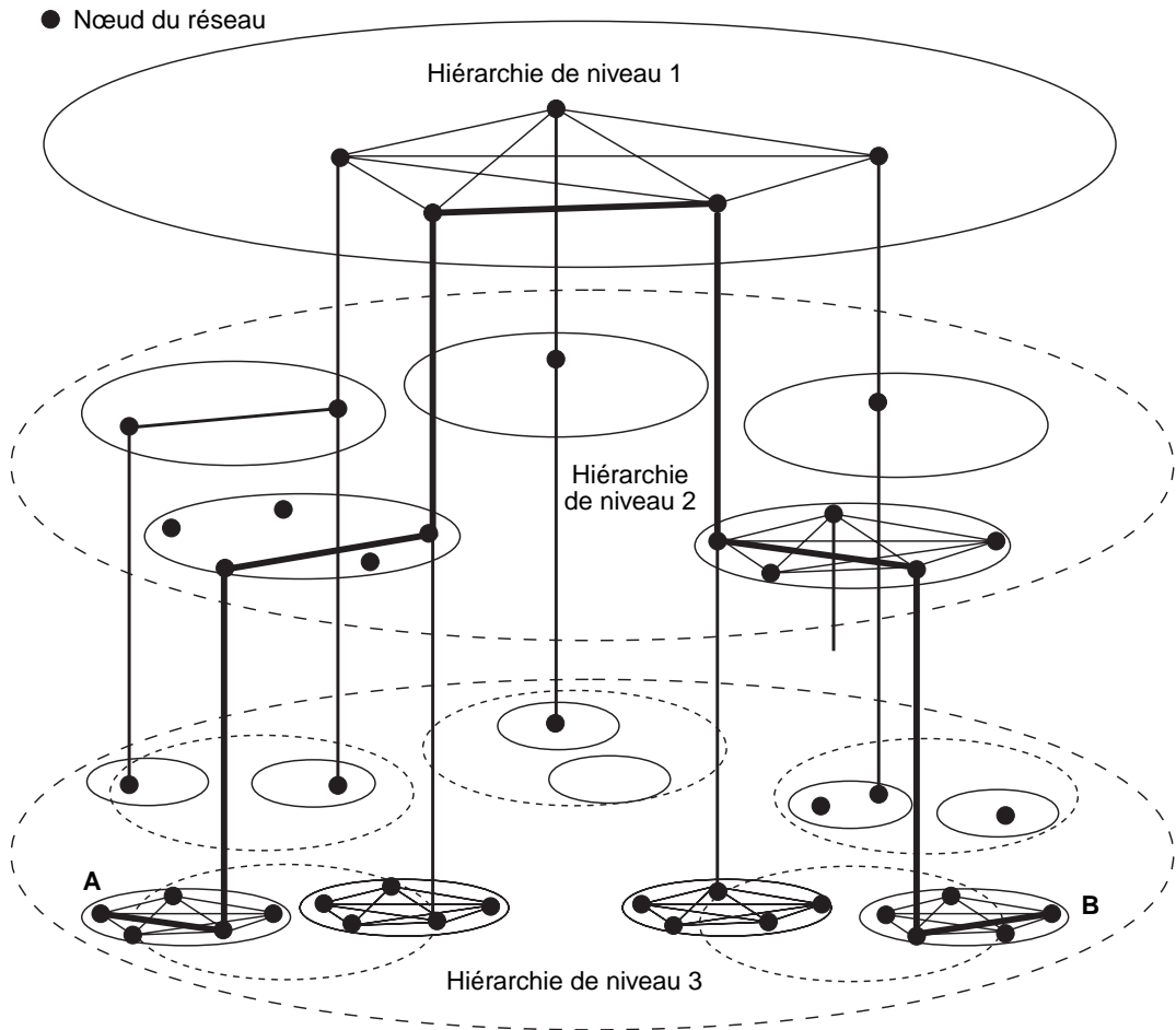
Figure 17.21 Hiérarchie de réseau à trois niveaux
