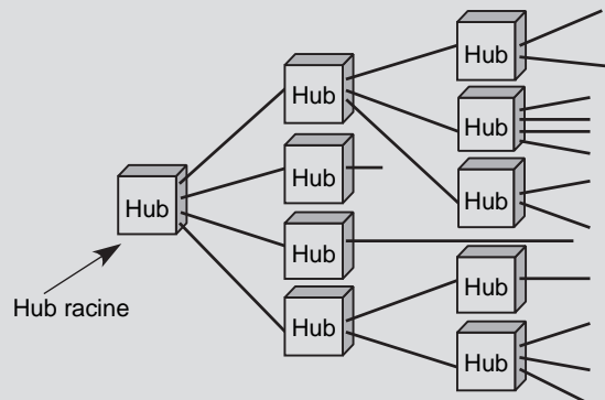
Figure 16.11 Architecture d'un réseau Starlan
