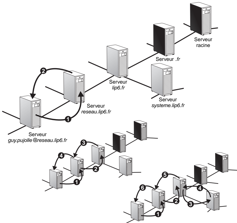
Figure 18.7 Fonctionnement du DNS
