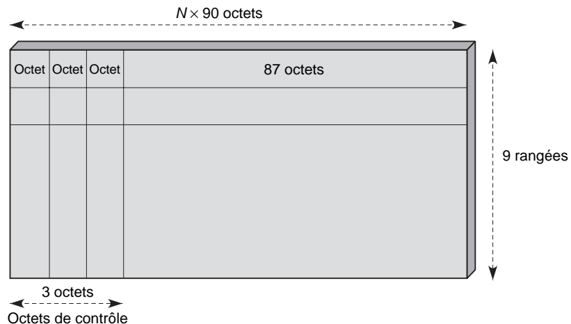
Figure 14.5 Trame SONET STS-N
