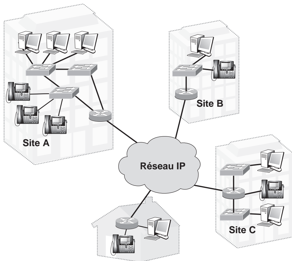
Figure 29.16 Réseau d'entreprise multisite
