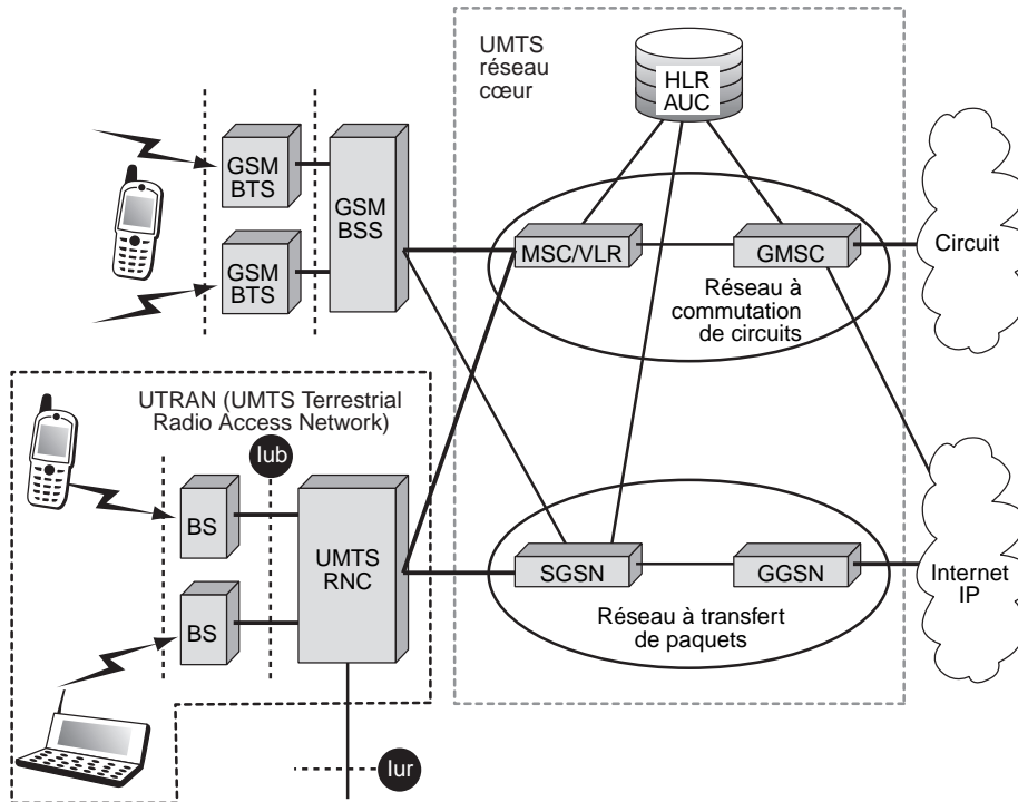
Figure 43.3 Architecture de la première génération de l'UMTS
