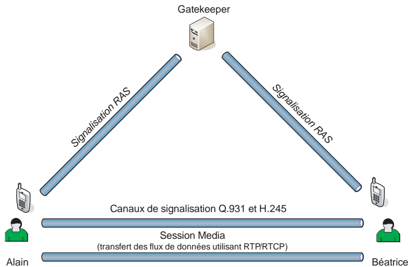
Figure 36.9 Signalisation en mode direct
