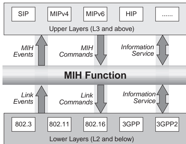
Figure 27.5 Emplacement de la fonction MIH dans la pile protocolaire IEEE 802.21
