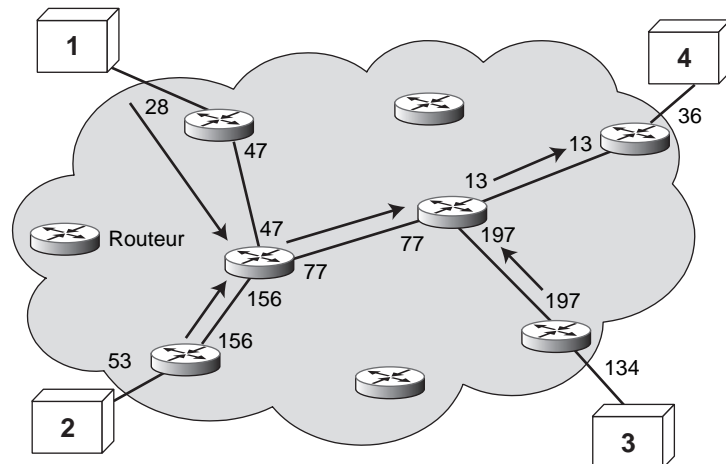
Figure 17.18 Classes d'équivalence (FEC) dans un réseau MPLS
