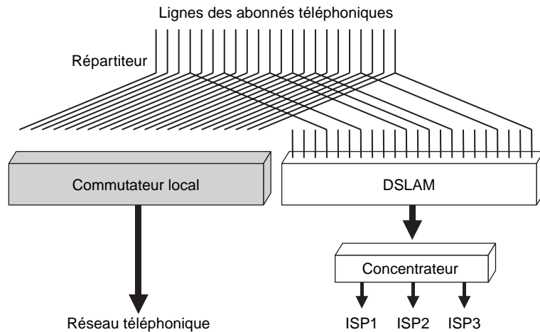
Figure 11.2 Positionnement d'un DSLAM
