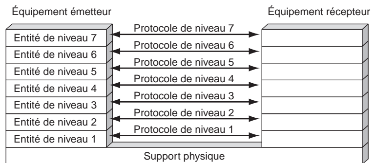
Figure 2.3 Architecture protocolaire d'un réseau à sept niveaux
