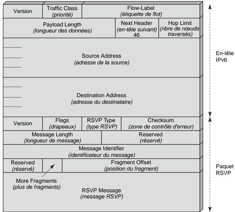
Figure 19.1 Format du message RSVP
