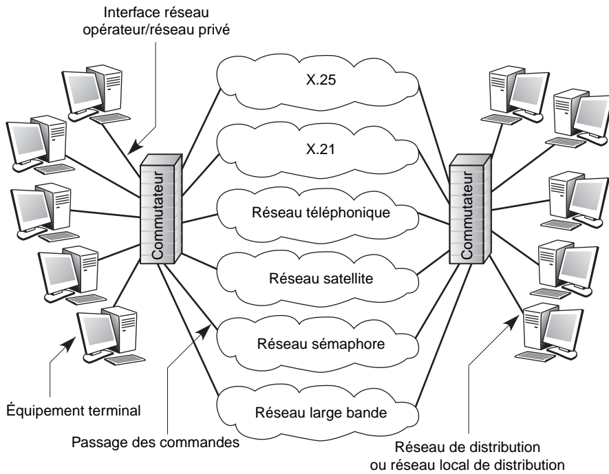
Figure 1.4 Extension du RNIS avec un réseau large bande
