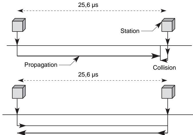
Figure 16.4 Temps maximal entre émission et réception d'une collision
