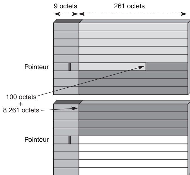
Figure 14.7 Transport d'un flux SDH à 140 Mbit/s
