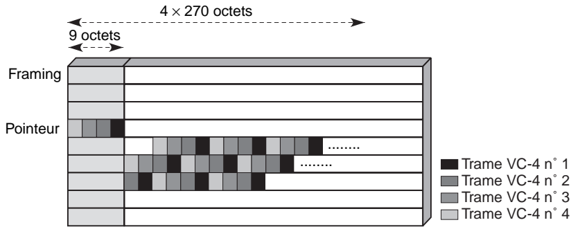
Figure 14.9 Multiplexage de containers VC-4 sur une trame STM-4
