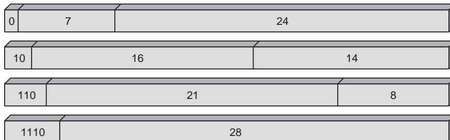
Figure 8.20 Classes d'adresses d'IPv4
