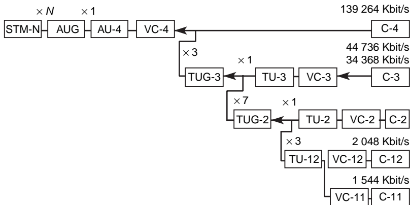
Figure 14.10 Hiérarchie SDH de l'ETSI
