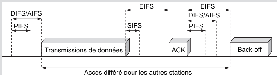
Figure 23.18 Les relations entre les différents temporisateurs
