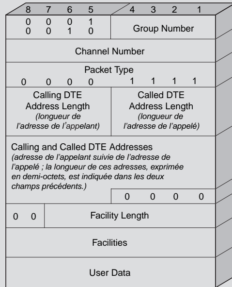
Figure 8.30 Paquet d'appel (CALL REQUEST)
