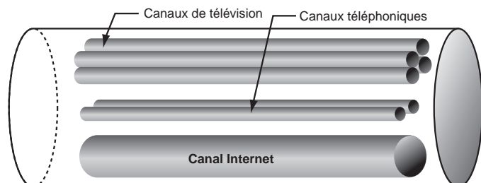
Figure 2.6 Multiplexage en fréquence dans le CATV
