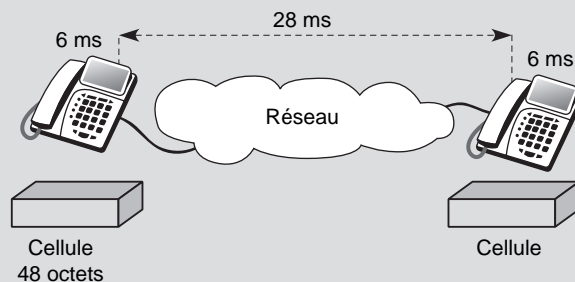
Figure 15.8 Contraintes de propagation de la parole téléphonique
