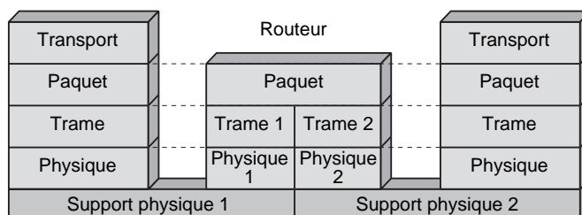
Figure 31.1 Architecture protocolaire d'un routeur
