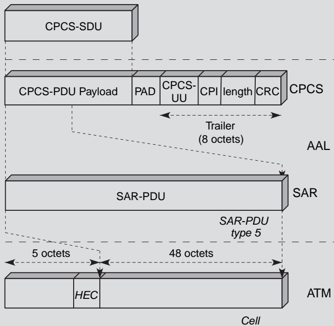
Figure 15.29 Empilement des protocoles dans la couche CS-5
