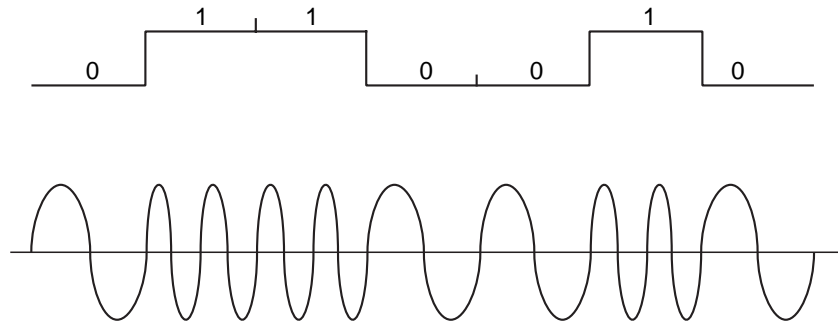
Figure 6.7 Modulation de fréquence
