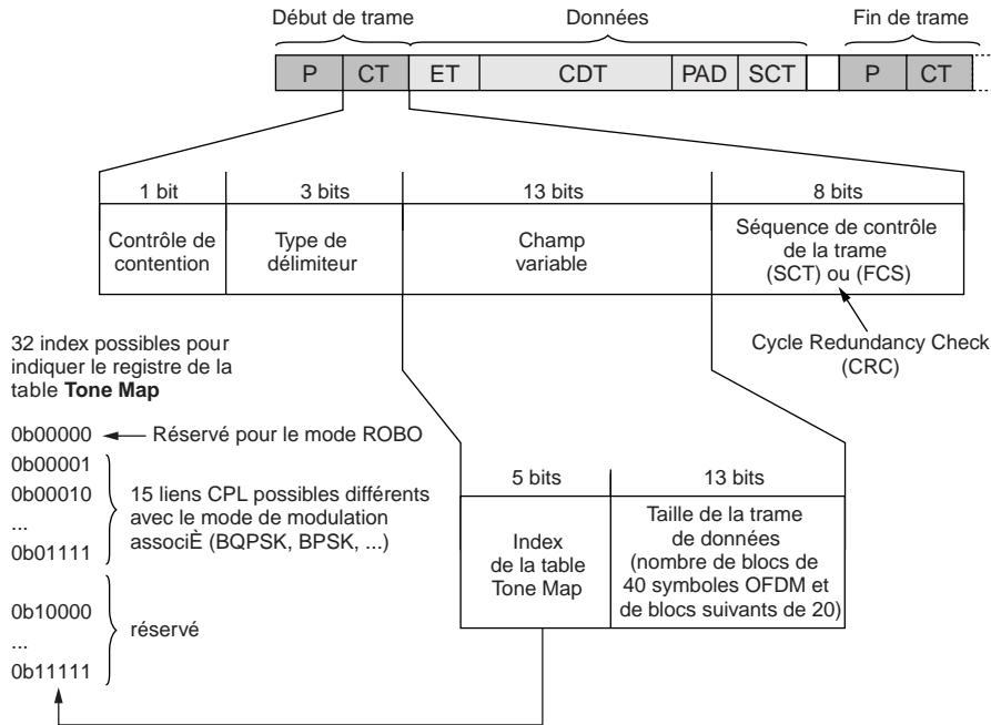
Figure 25.1 Champ Tone Map dans HomePlug 1.0
