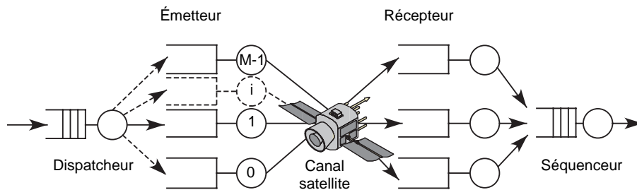
Figure 26.9 Protocole des sous-canaux virtuels
