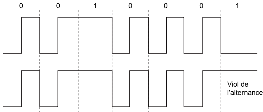
Figure 6.14 Principe du viol de polarité
