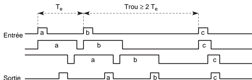
Figure 31.19 Retour en position de base
