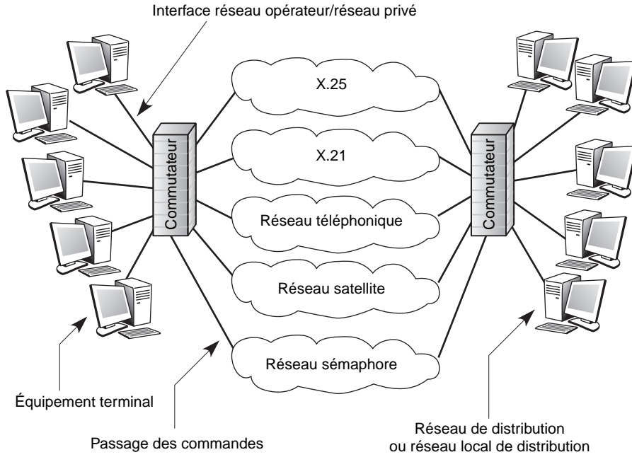
Figure 1.3 RNIS avec réseau sémaphore
