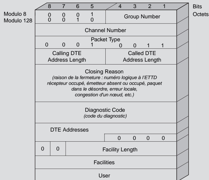
Figure 8.31 Format des trames de demande de libération et d'indication de libération
