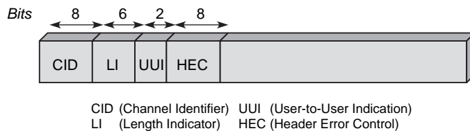
Figure 41.2 Minitrame de l'AAL2
