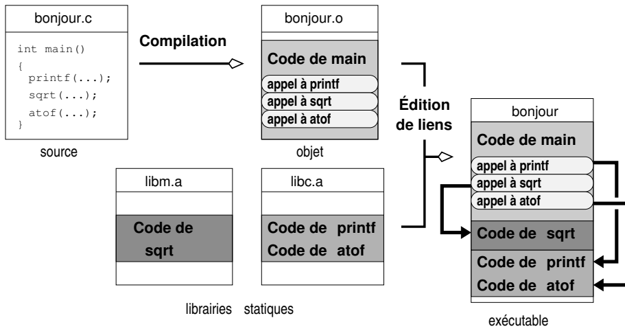
FIGURE 5.4 – Édition de liens statique.
