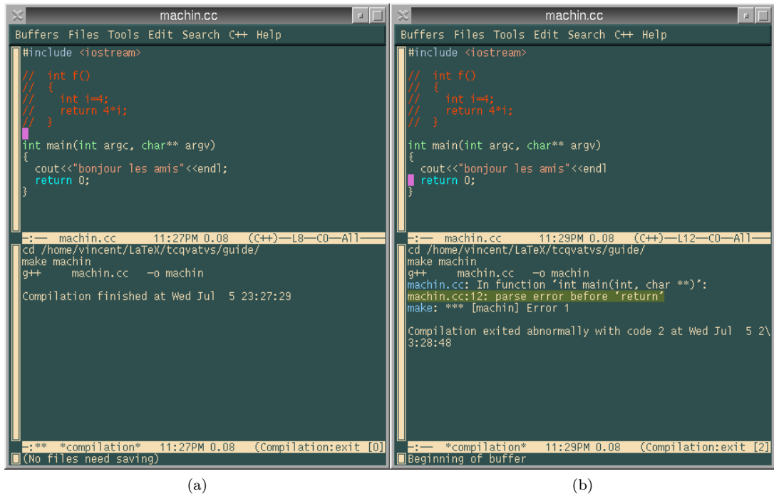
FIGURE 6.4 – Compilation dans Emacs
