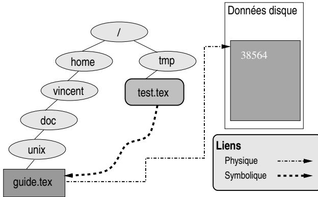
FIGURE 2.5 – Exemple de lien symbolique.
