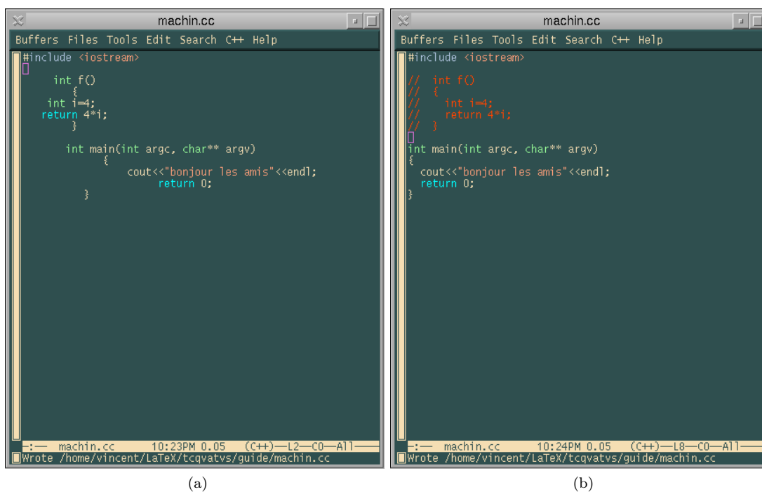
FIGURE 6.3 – Commentaires et indentation automatique : pour passer de la figure (a) à la figure (b), on a appelé la fonction M-x indent-region après avoir sélectionné le buffer entier ; puis après avoir sélectionné le corps de la fonction f() , on a fait appel à la commande M-x comment-region pour commenter son code.
